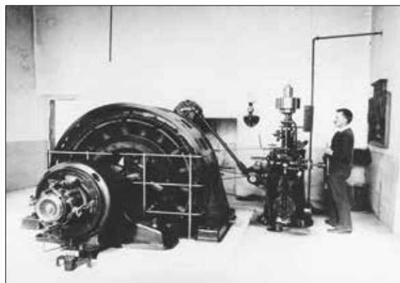
Strojnica z generatorjem elektrarne Pustnik z Ožboltom Ježem, okoli leta 1940
